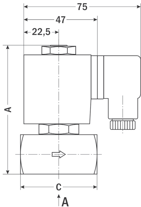
Вид А
