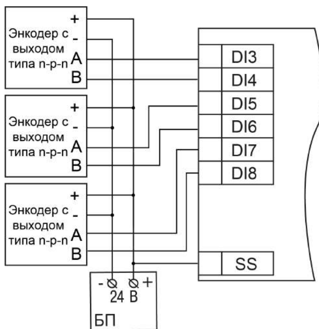
Рисунок 5.8 – Подключение энкодеров п-п-п
