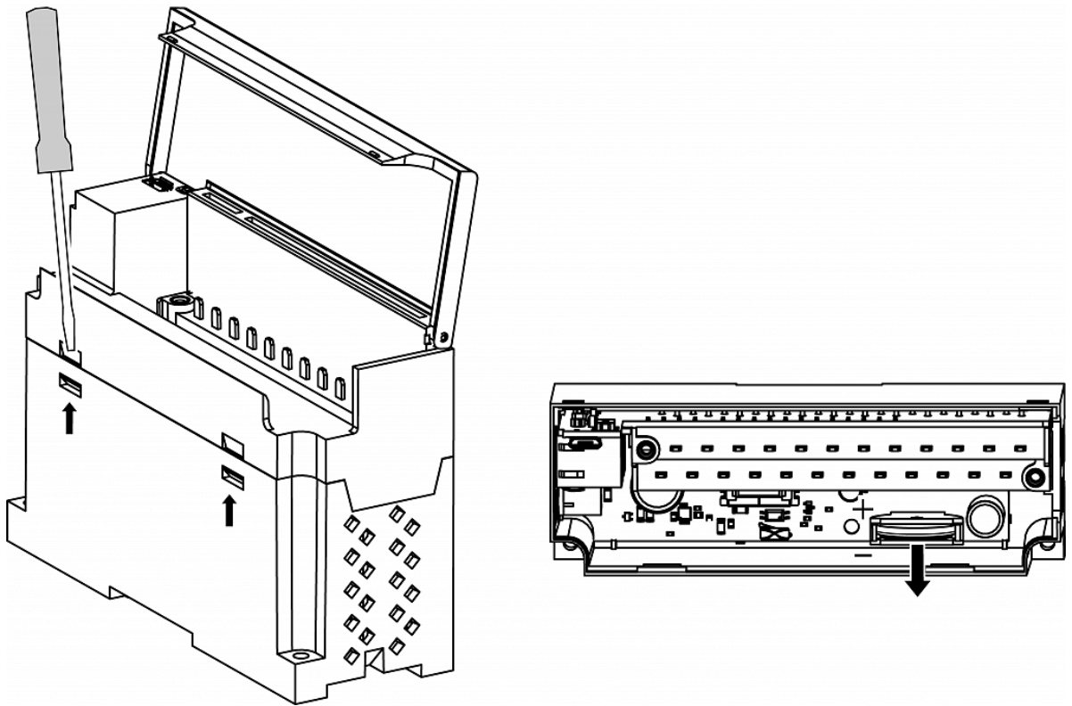
Рисунок 8.2 – Замена батареи
