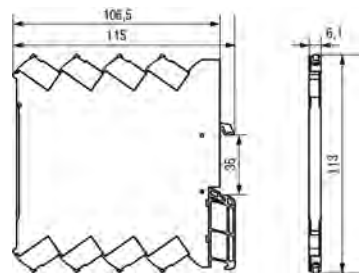
Рисунок 6.1 – Габаритный чертеж прибора
