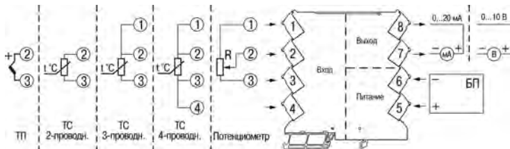
Рисунок 6.3 – Подключение прибора
