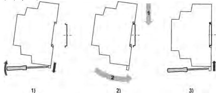
Рисунок 1 – Установка прибора
