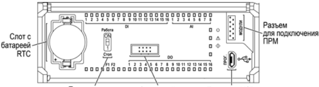
Рисунок 9 – Лицевая панель под крышкой
