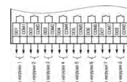
Рисунок 4 – Схема подключения нагрузок к ВЭ типа «Р»
