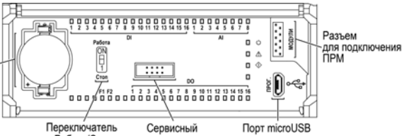
Рисунок 9 – Лицевая панель под крышкой
