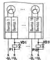
Рисунок 4 – Схема подключения нагрузок к ВЭ типа «К»
