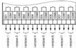
Рисунок 9 – Схема подключения нагрузок к ВЗ типа «Р»
