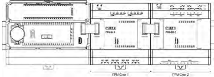
Рисунок 12 – Расположение модулей расширения на шине
