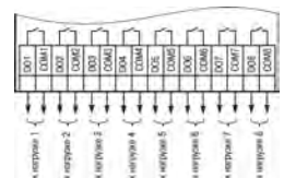
Рисунок 9 – Схема подключения нагрузок к ВЗ типа «Р»
