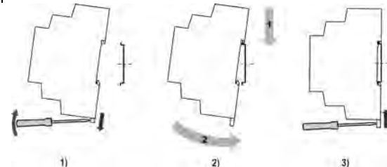
Рисунок 1 – Монтаж прибора
