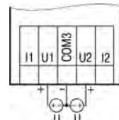
Рисунок 6 – Подключение датчиков с выходом в виде напряжения
