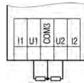
Рисунок 4 – Подключение резистивных датчиков
