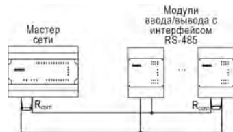
Рисунок 11 – Типовая схема подключения в режиме Master
