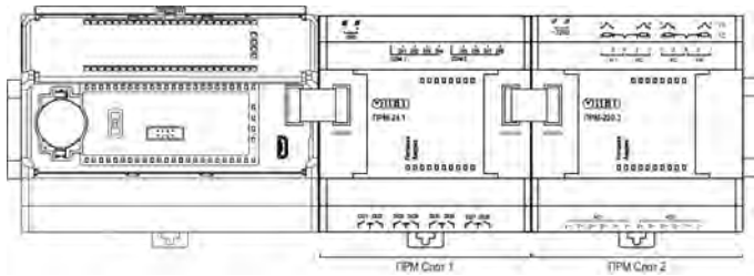
Рисунок 12 – Расположение модулей расширения на шине
