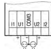
Рисунок 6 – Подключение датчиков с выходом в виде напряжения
