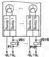
Рисунок 9 – Схема подключения нагрузок к ВЗ типа «К»
