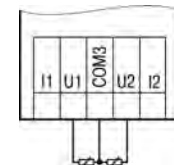
Рисунок 3 – Подключение ТС к AI
