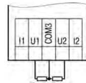
Рисунок 4 – Подключение резистивных датчиков
