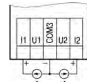
Рисунок 5 – Подключение датчиков с выходом в виде тока
