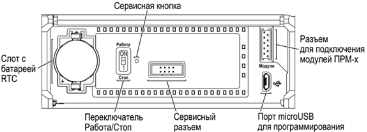
Рисунок 9 – Лицевая панель под крышкой
