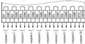
Рисунок 4 – Схема подключения нагрузок к ВЭ типа «Р»
