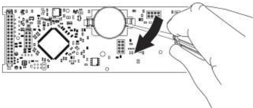
Рисунок 8.4 – Вид на обратную сторону верхней платы
