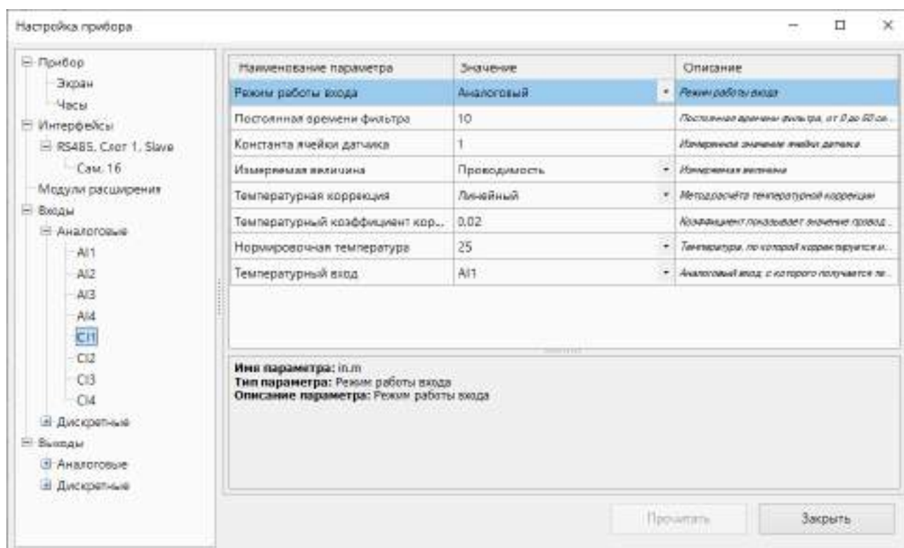
Рисунок 4.4 – Настройка кондуктометрического входа
