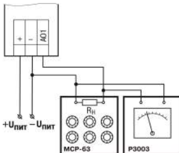
Рисунок Б.7 – Схема подключения к ВЭ для юстировки сигналов типа «4...20 мА» (R н < 300 Ом)
