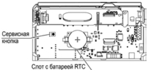
Рисунок 15 – Под лицевой панелью
