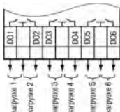
Рисунок 9 – Схема подключения ВЭ типа «Р»
