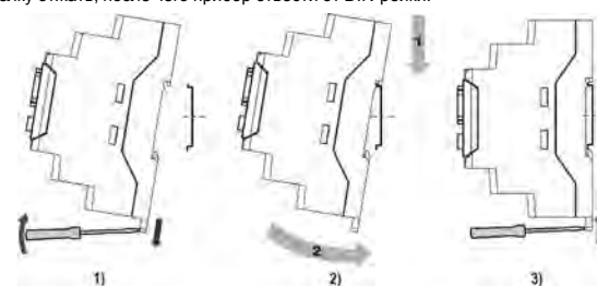
Рисунок 2 – Монтаж прибора
