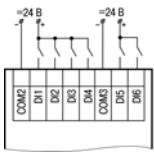
Рисунок 3 – Подключение к дискретным входам датчиков типа «сухой контакт» для сигналов =24 В
