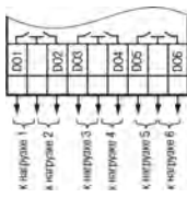
Рисунок 10 – Схема подключения ВЭ типа «Р»
