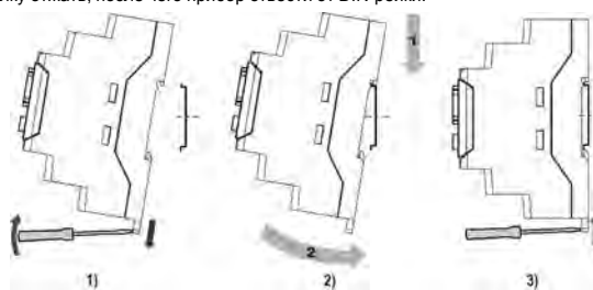
Рисунок 2 – Монтаж прибора
