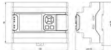
Рисунок 1 – Габаритные размеры прибора
