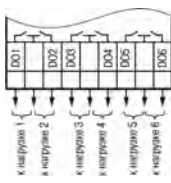
Рисунок 10 – Схема подключения ВЭ типа «Р»
