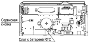
Рисунок 16 – Под лицевой панелью
