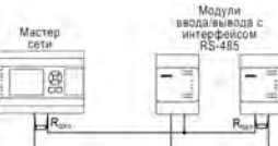
Рисунок 14 – Типовая схема подключения в режиме Master
