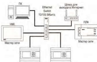
Рисунок 15 – Подключение по схеме «Звезда»
