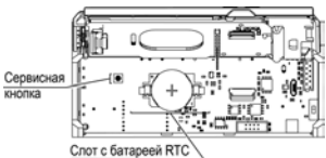
Рисунок 18 – Под лицевой панелью
