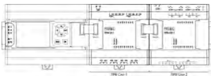
Рисунок 16 – Расположение модулей расширения на шине
