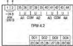
Рисунок 3 – Назначение контактов клеммника
