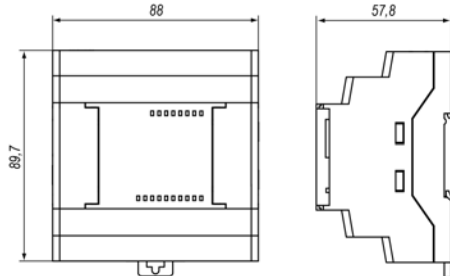
Рисунок 2 – Габаритные размеры
