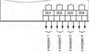
Рисунок 12 – Схема подключения нагрузки к ВЭ типа «Р»
