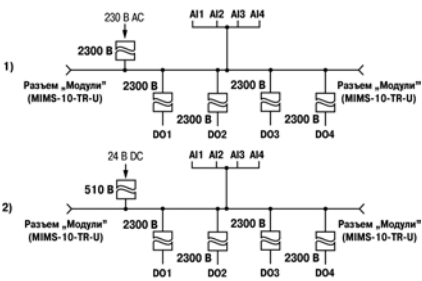
Рисунок 4 – Схемы гальванической развязки (1) 230 В и (2) 24 В модификаций
