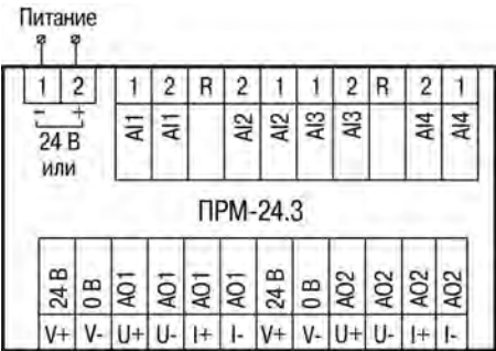
Рисунок 5.2 – Назначение контактов клеммника прибора с питанием 24 В
