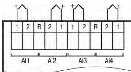
Рисунок 5.6 – Подключение ТП к AI ПРМ-х.3
