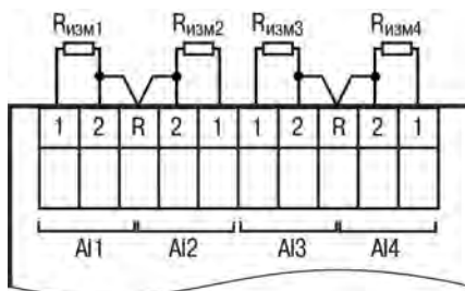
Рисунок 5.9 – Подключение резистивных датчиков
