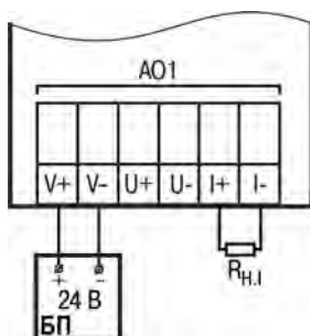
Рисунок 5.10 – Схема подключения к АО ПРМ-х.3 типа И (0(4)...20 мА)
