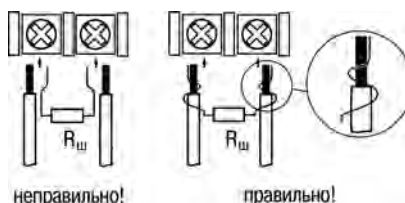
Рисунок 5.8 – Подключение шунтирующего резистора
