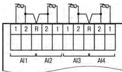
Рисунок 5.5 – Подключение ТС к аналоговым входам (AI) ПРМ-х.3
