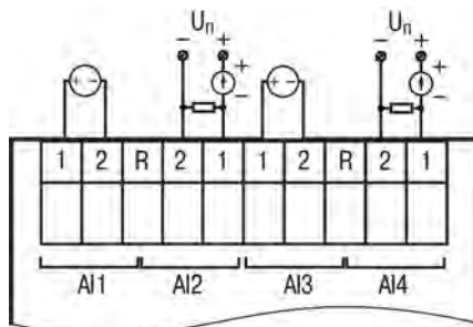
Рисунок 5.7 – Подключение датчиков с выходом в виде напряжения (к AI1 и AI3) и с выходом в виде тока (к AI2 и AI4)
