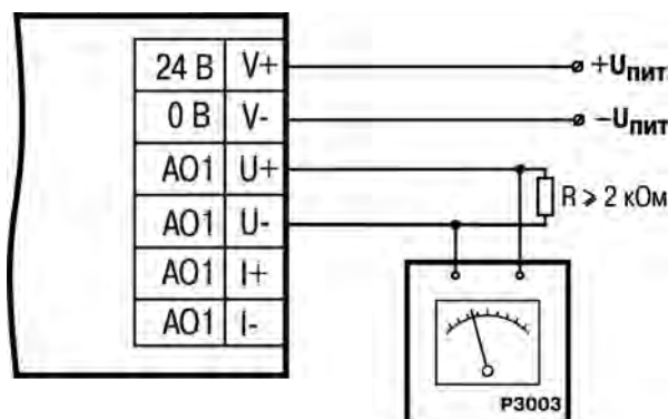
Рисунок 8.9 – Схема подключения нагрузки к ВЭ типа У
