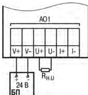
Рисунок 5.11 – Схема подключения к АО ПРМ-х.3 типа У
