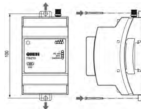
Рисунок 3 – Крепление винтами
