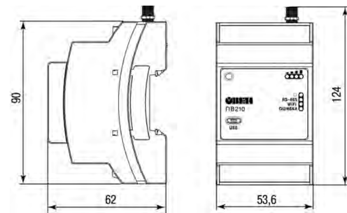
Рисунок 2 – Габаритные размеры
