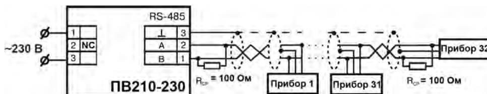
Рисунок 5.2 – Схема подключения ПВ210 с номинальным напряжением питания 230 В переменного тока
