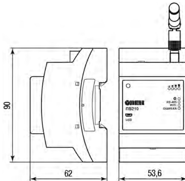
Рисунок 4.1 – Габаритные размеры
