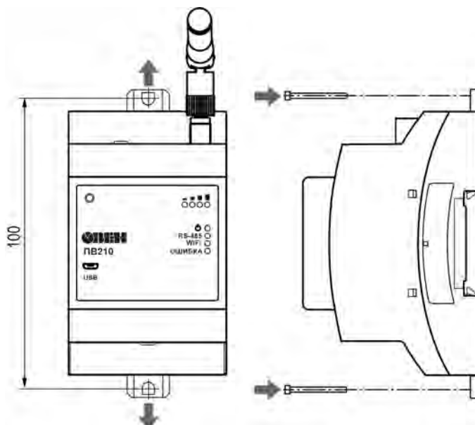
Рисунок 4.2 – Крепление винтами
