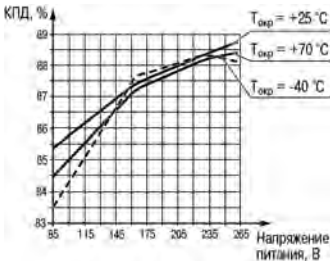
Рисунок 7 - График зависимости КПД от напряжения питания и температуры окружающей среды
