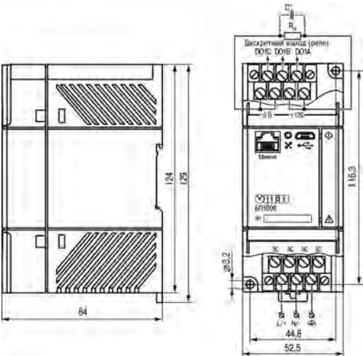
Рисунок 1 - Габаритные, установочные размеры и подключение прибора
