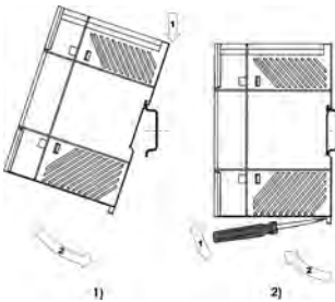
Рисунок 2 - Монтаж (1) и демонтаж (2) прибора
