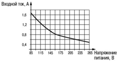
Рисунок 5 - График зависимости входного тока от напряжения питания
