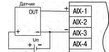
Рисунок 6 – Схема подключения датчиков с унифицированным выходным сигналом –50...50 мВ и –1...1 В по трехпроводной схеме
