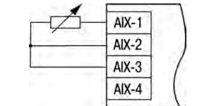
Рисунок 9 – Схема подключения датчиков типа 0...2 кОм и 0...5 кОм
