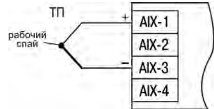
Рисунок 5 – Схема подключения TP
