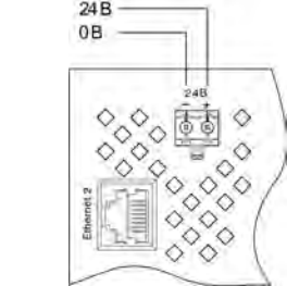
Рисунок 2 – Подключение питания
