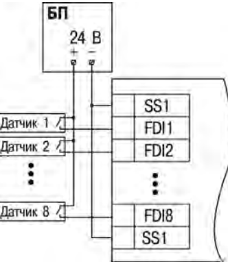
Рисунок 11 – Схема подключения контактных датчиков к дискретным входам FDI1–FDI8
