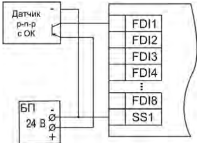
Рисунок 12 – Подключение транзисторов типа р-п-р
