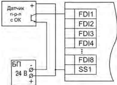
Рисунок 13 – Подключение транзисторов типа п-р-п
