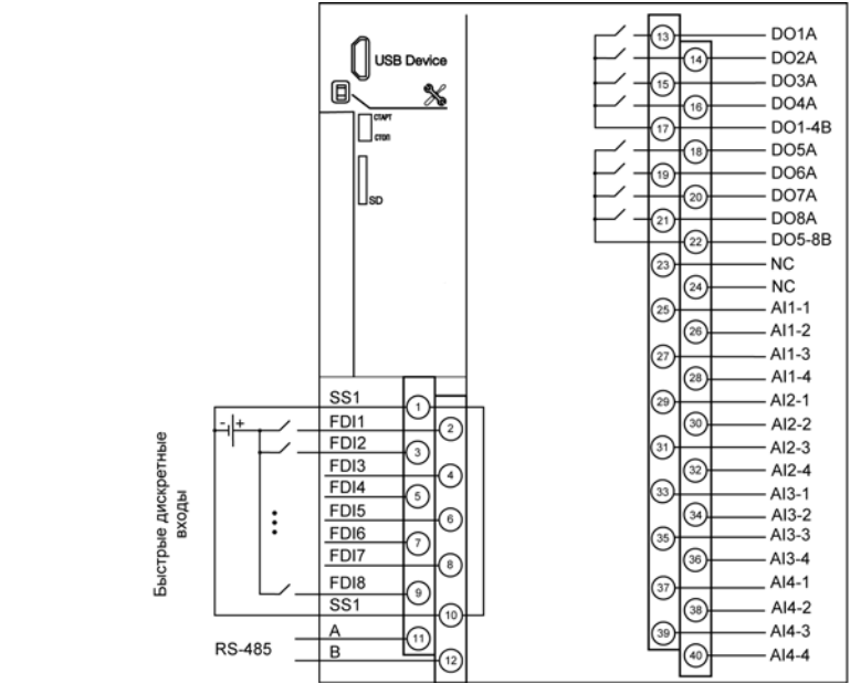
Рисунок 3 – Назначение контактов клеммника
