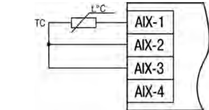
Рисунок 4 – Схема подключения TC по трехпроводной схеме
